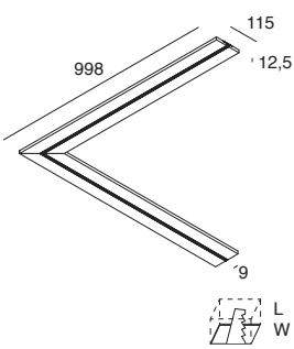
PROFILO ANGOLARE 90° 90° CORNER PROFILE
