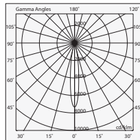
BEAM 14°
