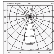
BEAM 34°
