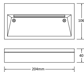
APPLIQUE - 102801.94
