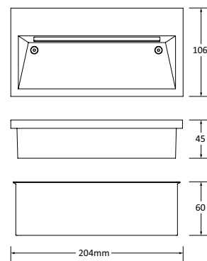
INCASSO/RECESSED - 102802.94
